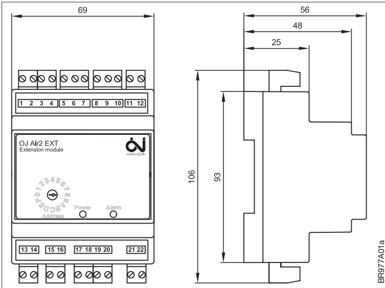
Fig. 1 - Dimensions
